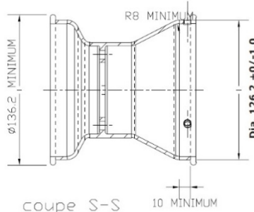
coupe S-S
